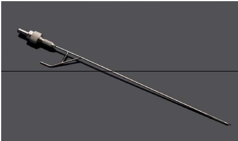
Injektionskanüle mit Flüssigkeits- oder Druckluftzufuhr mit SMA-Anschluss für faseroptische Strahlführungssysteme
